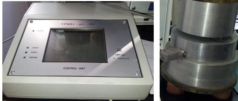
Fot. 4. Aparatura TPMU- a \lambda -20 do określenia przewodności cieplnej i dyfuzyjności niemetalicznych materiałów stałych, od lewej: kontroler, jednostka grzewcza
